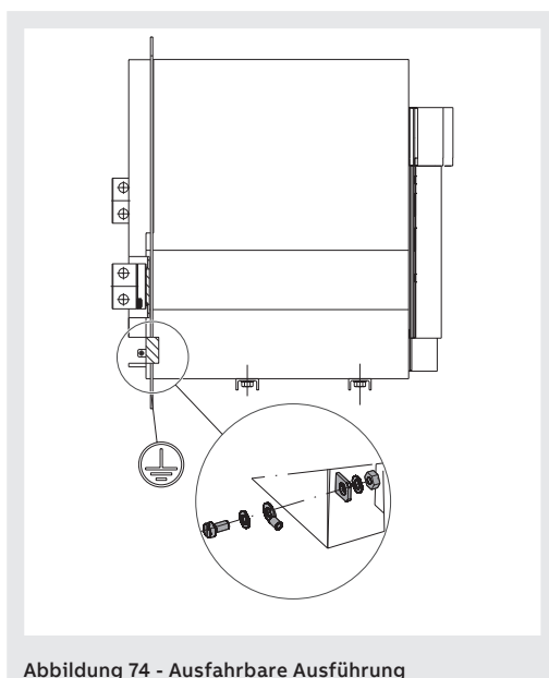
Abbildung 74 - Ausfahrbare Ausführung
