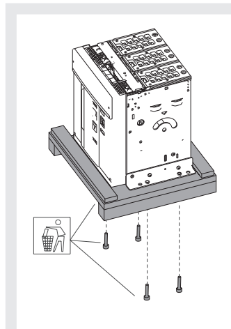
Abbildung 10 Fester Leistungsschlater
