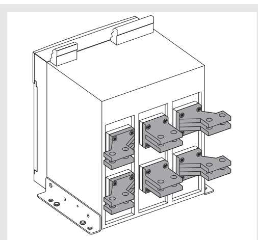
Abbildung 59 SHR - Rückseitig horizontal mit V-Form IEC (E2.2)
