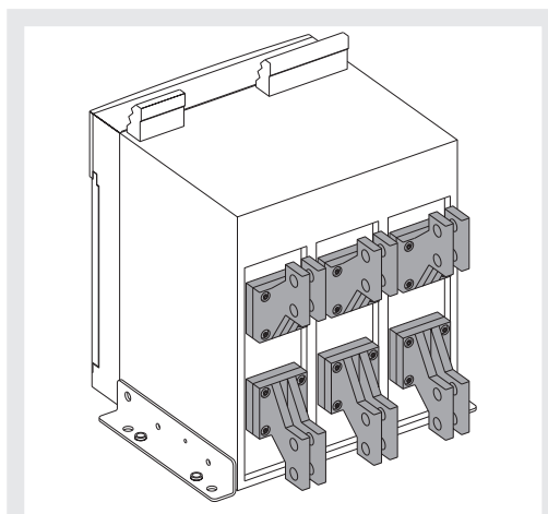
Abbildung 60 SVR - Rückseitig vertikal mit V-Form IEC (E2.2)
