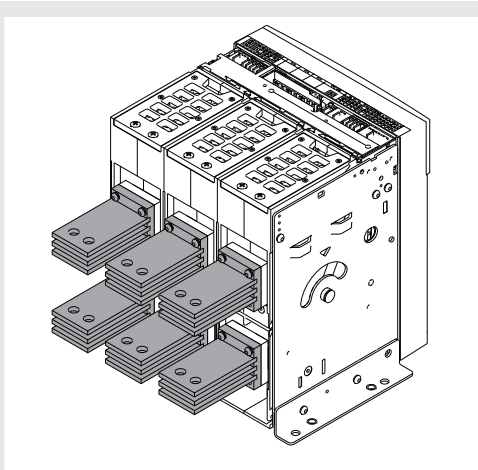
Figura 62 HR - Posteriori orizzontali UL Listed
