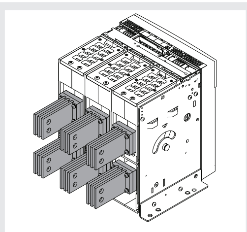
Figura 63 VR - Posteriori verticali UL Listed
