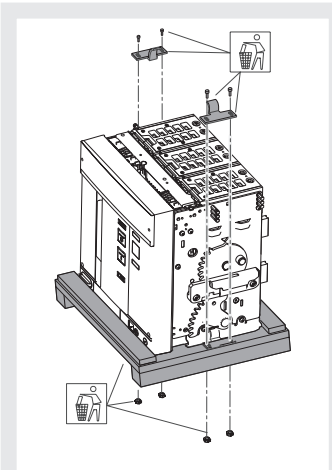
Figura 11 Parte mobile IEC
