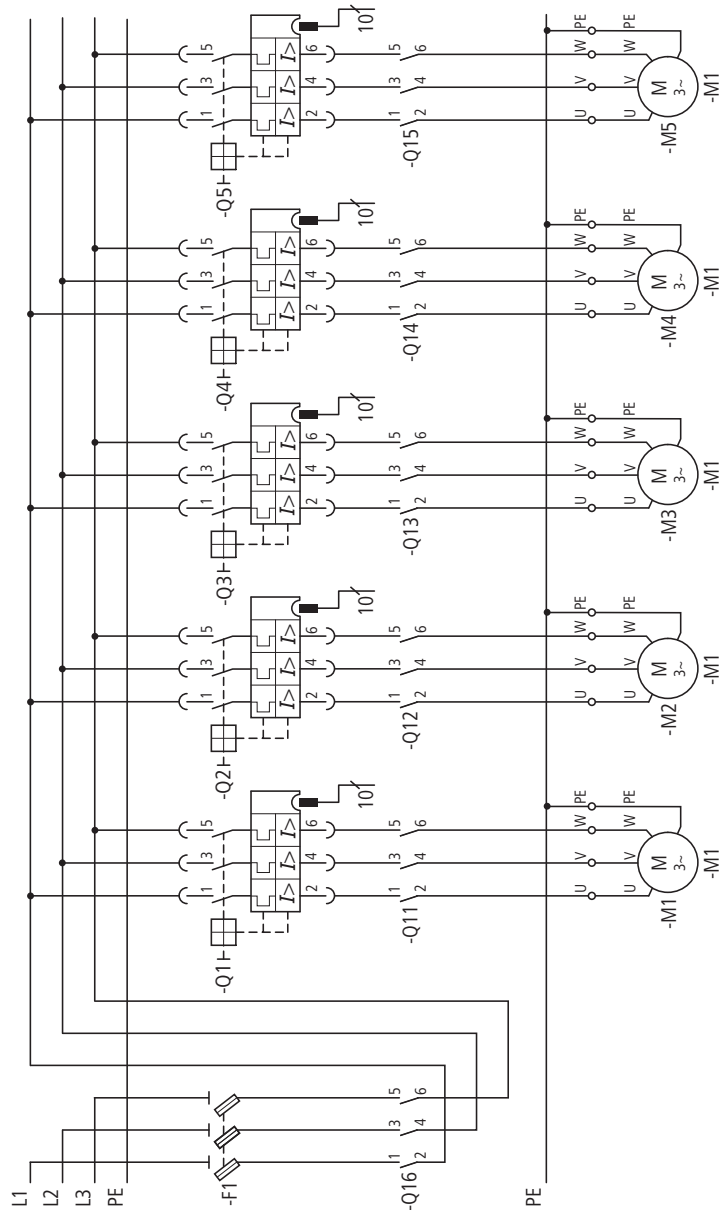
Figura 45: Circuito principale per disinserzione ridondante di gruppi di azionamenti
