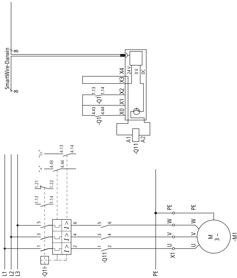
Figura 12: Schema elettrico dell'aviatore diretto
