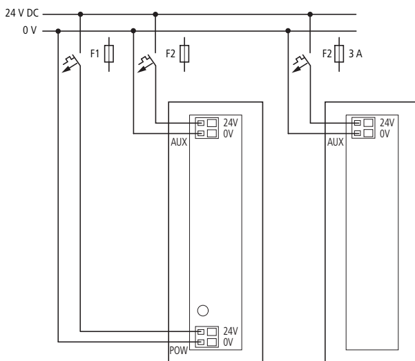
Figura 4: Sezioni di collegamento
