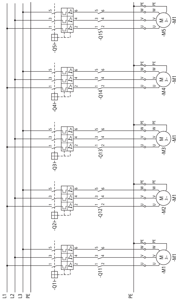
Figura 16: Circuito principale per disinserzione di sicurezza
