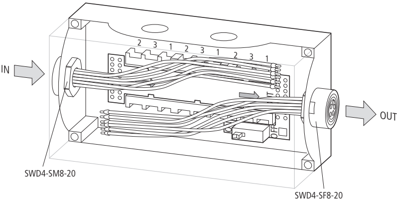
Figura 29: Collegamento mediante connettore
