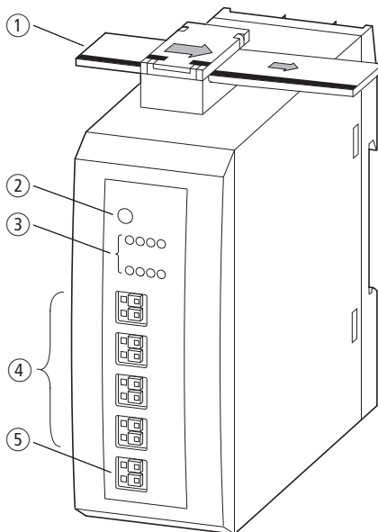
Figura 5: Collegamenti del power feeder EU5E-SWD-8DX
