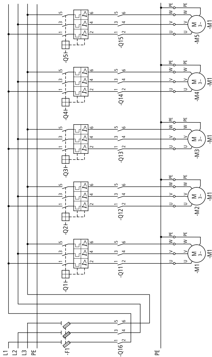
Figura 18: Circuito principale per disinserzione ridondante
