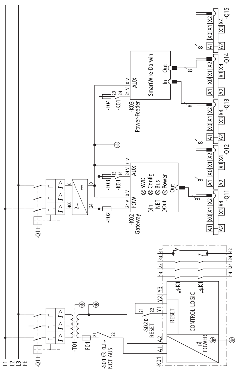
Figura 15: Circuito di alimentazione per disinserzione di sicurezza
