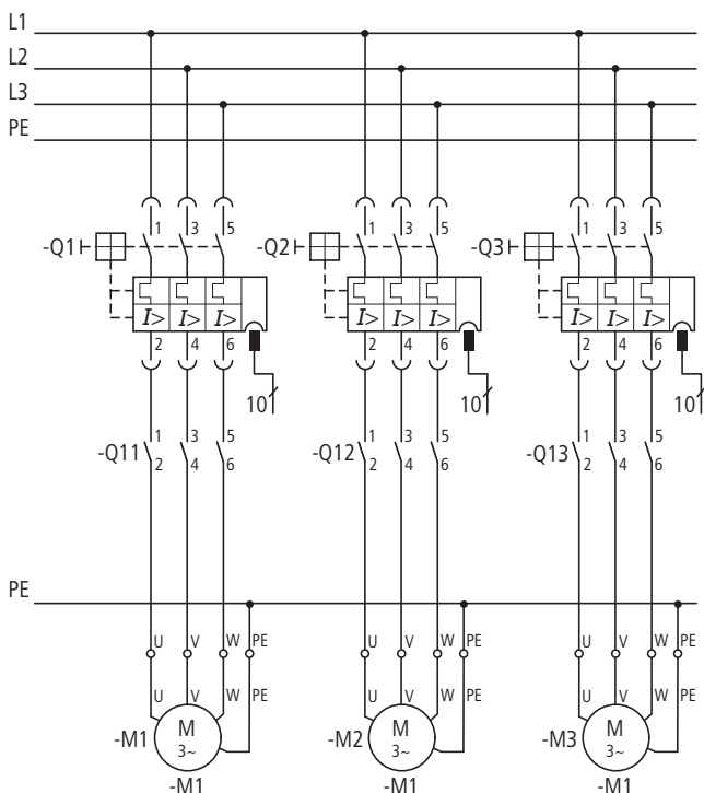
Figura 39: Circuito principale per disinserizione di sicurezza di un singolo azionamento
