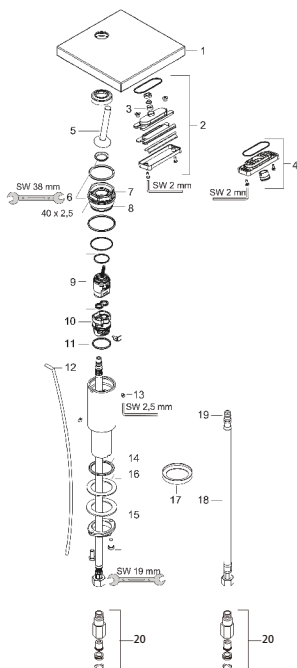
部品リスト
