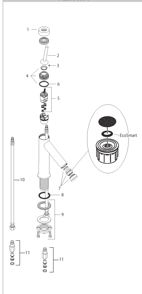
部品リスト
