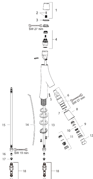
部品リスト
