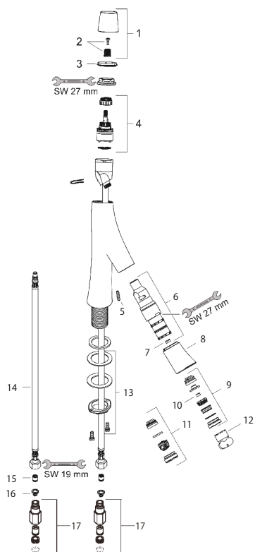
製品分解図
