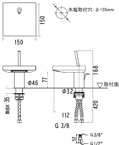
完成図
