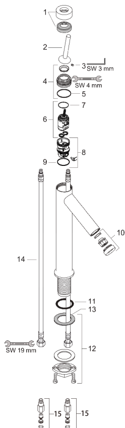
部品リスト
