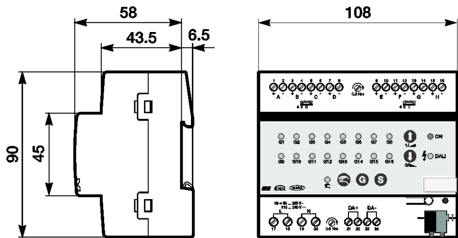
2.1.3 Rysunek wymiarowy DLR/S 8.16.1M
