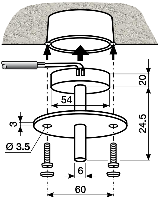
Rysunek wymiarowy LF/U 2.1
