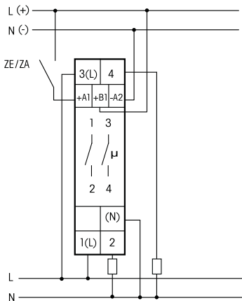
mit Kontaktschaltung im Nulldurchgang
