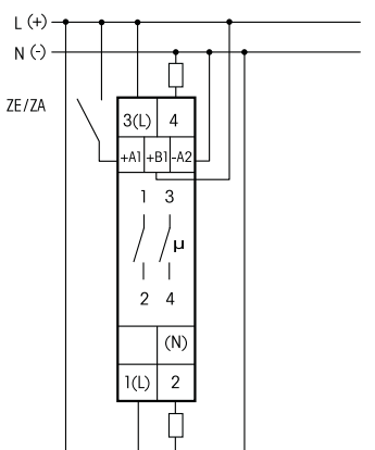
ohne Kontaktschaltung im Nulldurchgang
