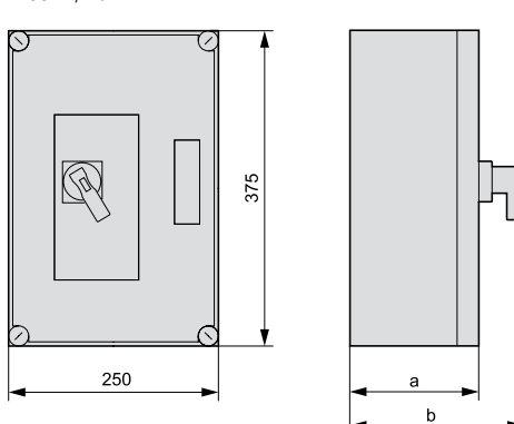
MCCB.../I43E-...
