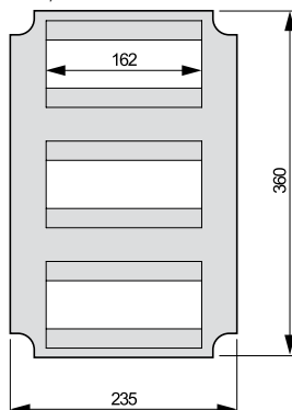
GA-0/I43
