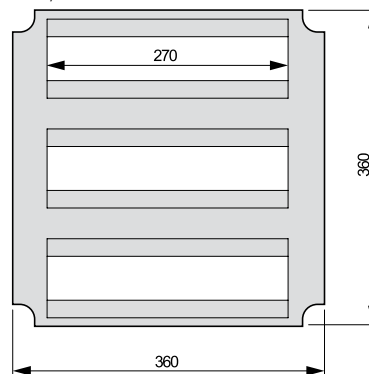
GA-0/I44
