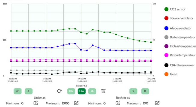
Signaalanalysator (trend)
