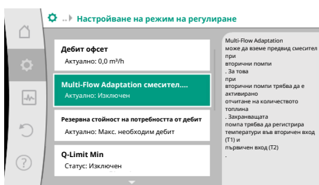
Fig. 59: Настройване на режим на регулиране: Multi-Flow Adaptation смесител
