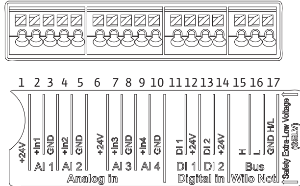
Fig. 20: Клемы за аналогови, цифрови входове и Wilo Net
