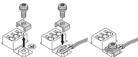
Fig. 22: Неподвижен захранващ кабел
