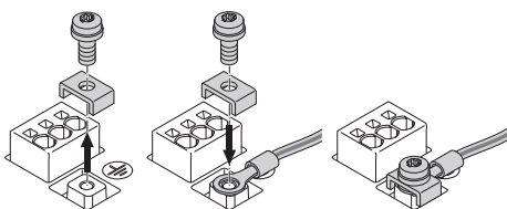
Fig. 21: Гъвкав захранващ кабел
