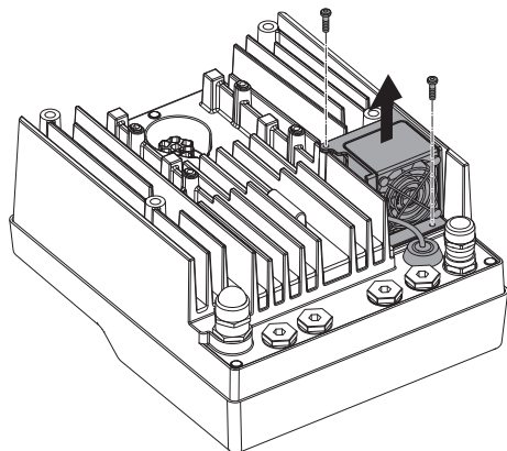
Fig. 110: Демонтаж на вентилатора на модула
