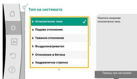
Fig. 41: Пример тип система „Отоплително тяло“
