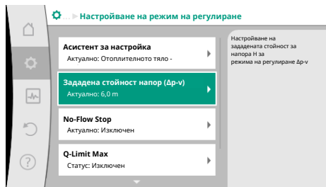
Fig. 70: Редактор за зададена стойност
