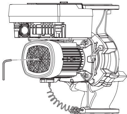
Fig. 5: Завъртане на вала
