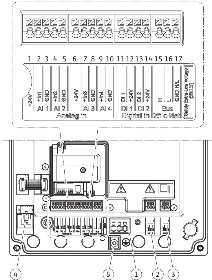
Fig. 19: Преглед клеми в модул
