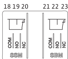
Fig. 23: Клеми за SSM и SBM
