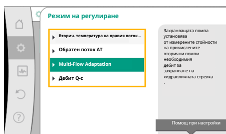
Fig. 55: Пример режим на регулиране „Multi-Flow Adaptation“
