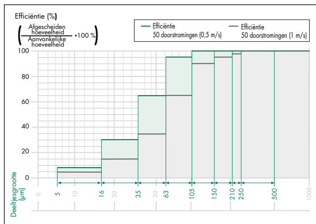
Proeven in het gespecialiseerde laboratorium van TNO - Science and Industry (NL)
