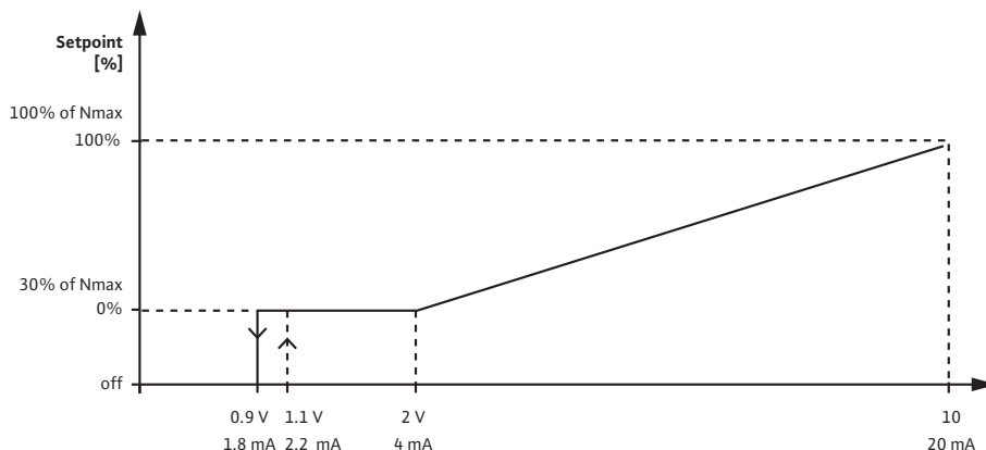
Fig. 36: Вход за зададена стойност 0 – 10 V или 0 – 20 mA
