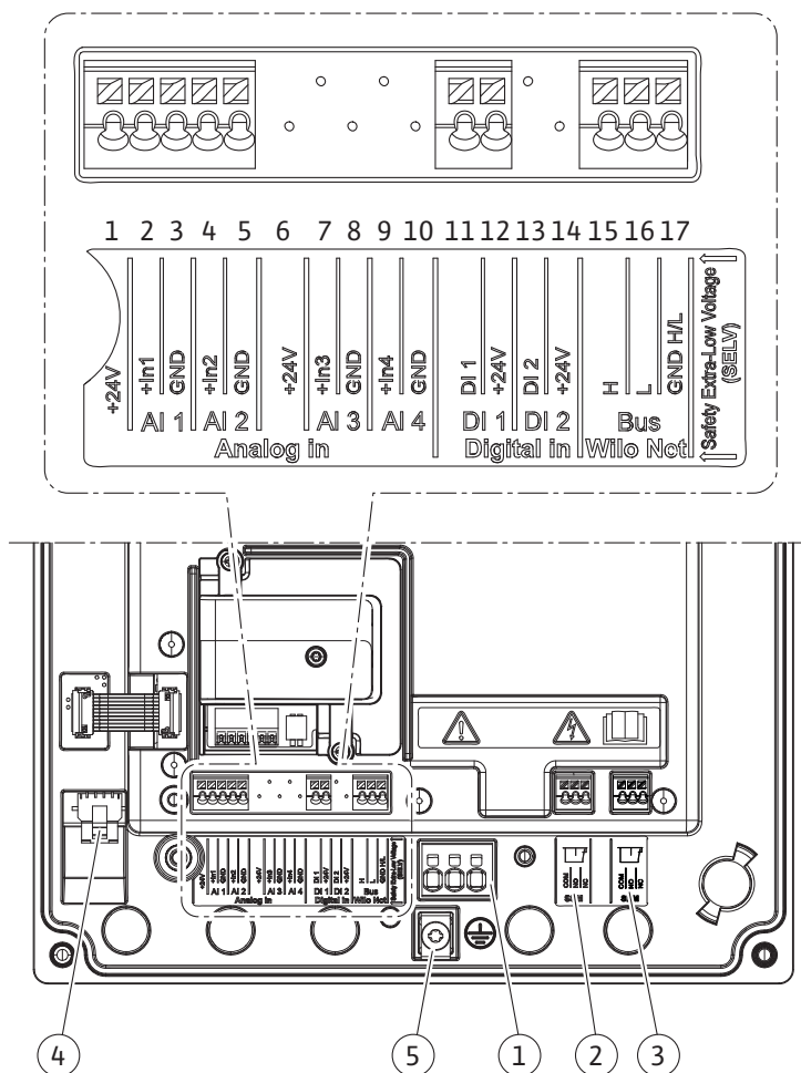
Fig. 11: Преглед клемни в модул
