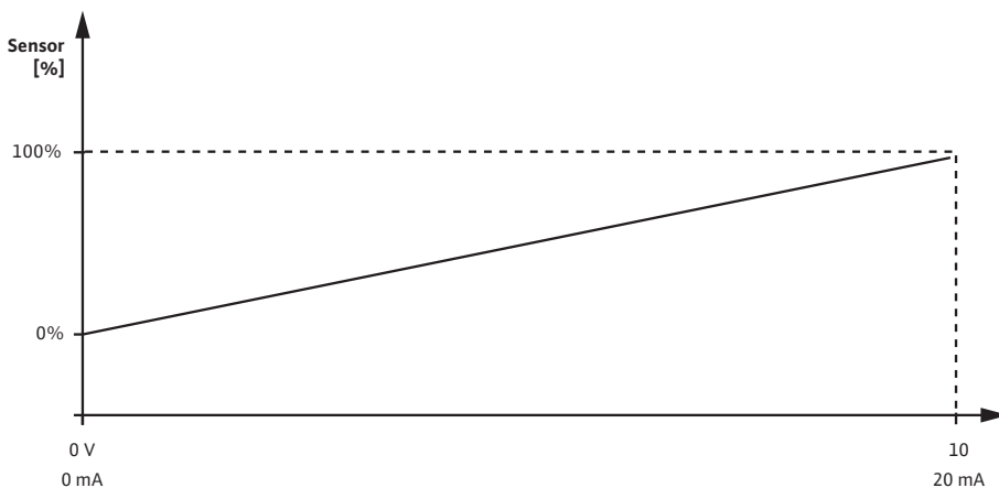
Fig. 38: Вход за датчик 0 – 10 V или 0 – 20 mA
