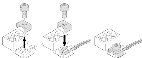
Fig. 14: Starre aansluitkabel
