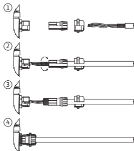
Fig. 16: Schermklem
