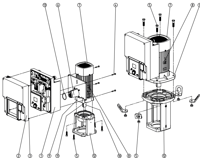
Fig. 1: Hoofdonderdelen
