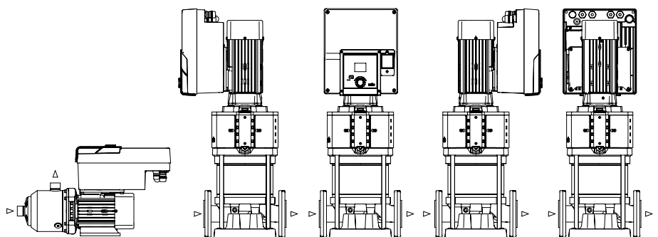
Fig. 4: Opstelling van de componenten bij levering
