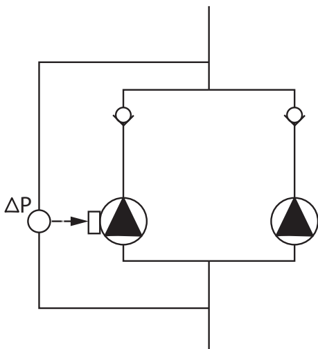
Fig. 9: Voorbeeld van de aansluiting van een verschildruksensor in een gezamenlijke verzamelbuis
