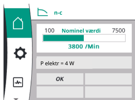
Fig. 24: Hovedmenu
