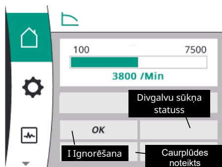
Fig. 26: Sākuma ekrāns: aktīvās ietekmes
