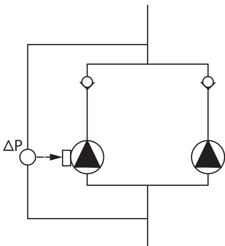
Fig. 9: Piemērs: relatīvā spiediena starpības sensora pieslēgums kopējā caurulē
