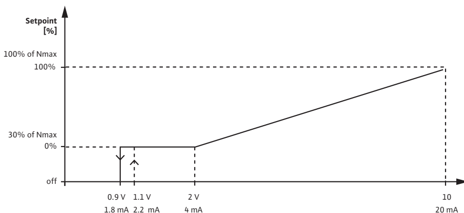
Fig. 36: Uzdotās vērtības ieeja 0–10 V vai 0–20 mA
