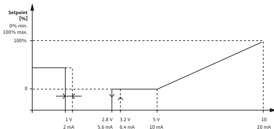
Fig. 37: Uzdotās vērtības ieeja 2–10 V vai 4–20 mA
