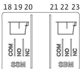
Fig. 15: SSM un SBM spaiļes
