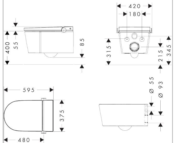
Maattekening
