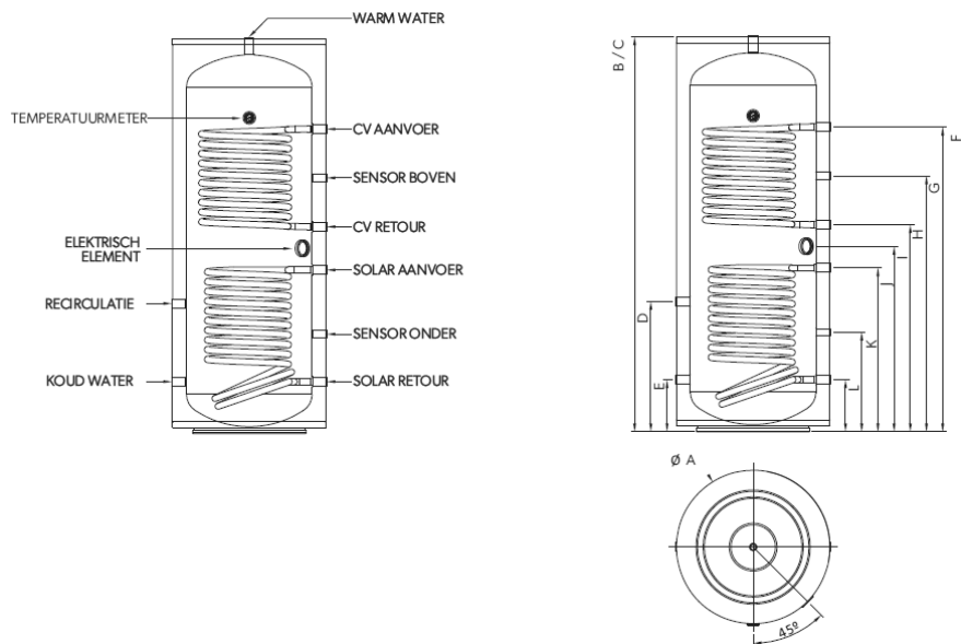
Figuur 2 Solar boiler
