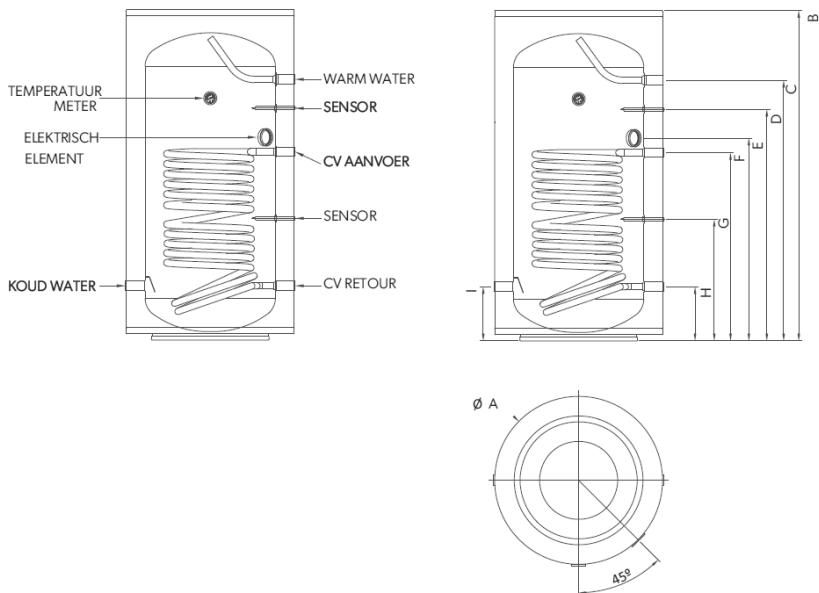
Figuur 4 Boiler t.b.v. warmtepomp verticaal MODUL-AIR
