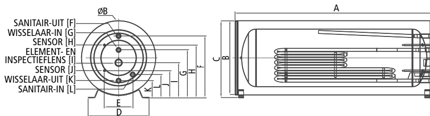
Figuur 6 Boiler t.b.v. warmtepomp horizontaal
