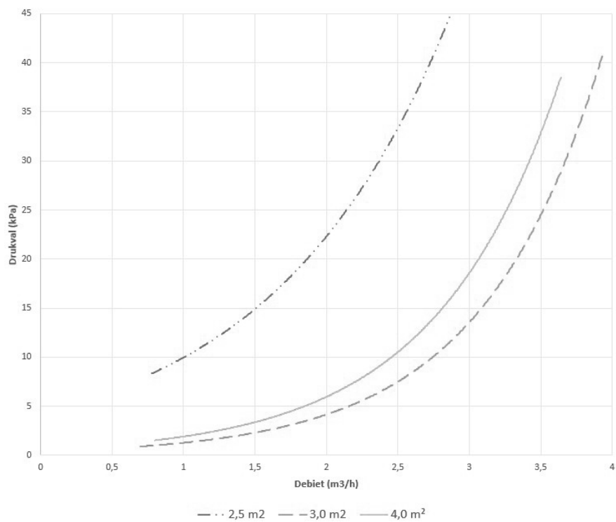
Figuur 9a Drukverlies warmtespiralen
