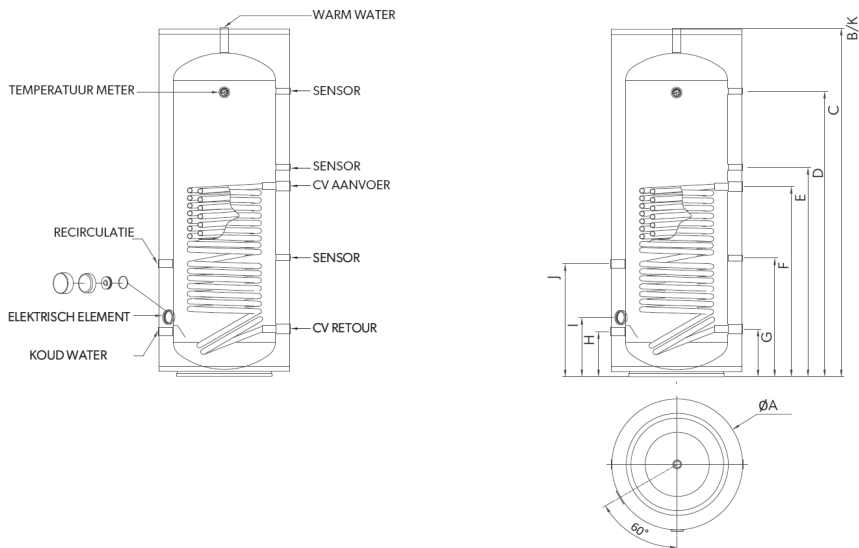
Figuur 3 Boiler t.b.v. warmtepomp verticaal
