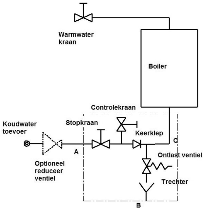
Figuur 12 Schema inlaatcombinatie
