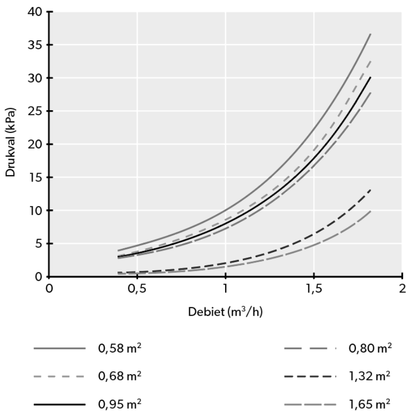
Figuur 9 Drukverlies warmtespiralen
