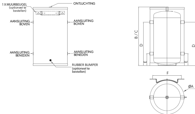
Figuur 8 Buffervat
