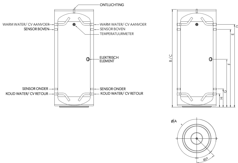
Figuur 7 Voorraadvat
