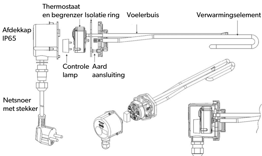
Figuur 17 Onderdelen van inschroefelement
