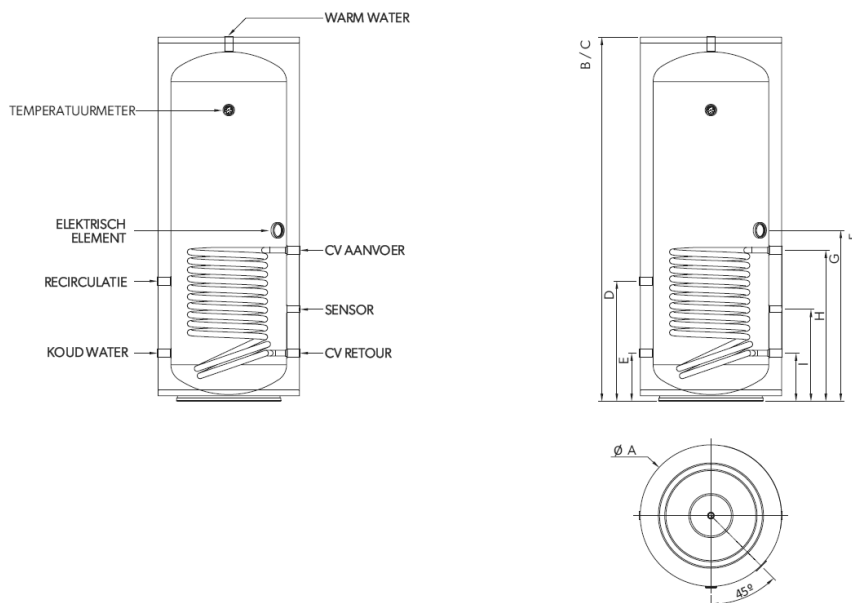
Figuur 1 Indirect verwarmde boiler
