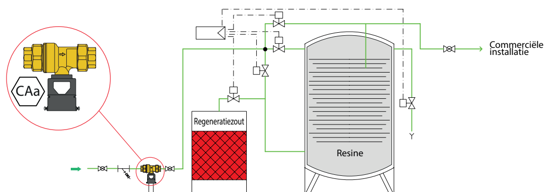
15. Waterverzachters voor commercieel gebruik (alleen met regeneratie met keukenzout) (cat. 3)
