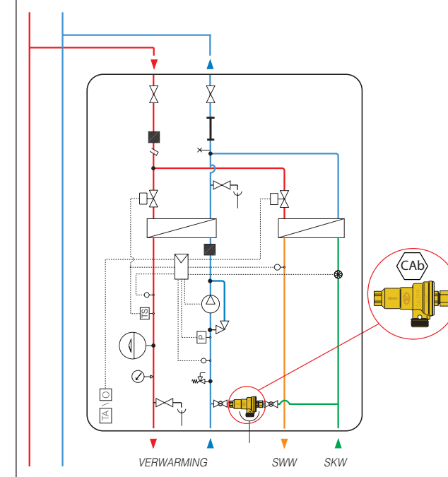
12. Vullen van het verwarmingscircuit in distributie-unit met gescheiden watervoorziening (cat. 3)
