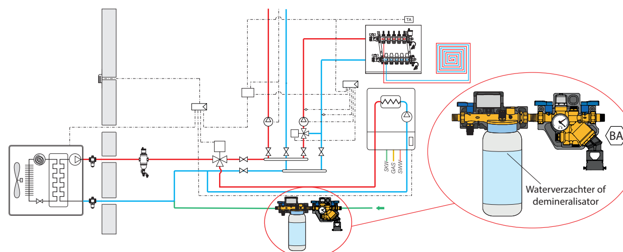
14. Vullen van gesloten circuits met doseerinrichtingen voor additieven zoals verzachters of demineralisators (cat. 4)
