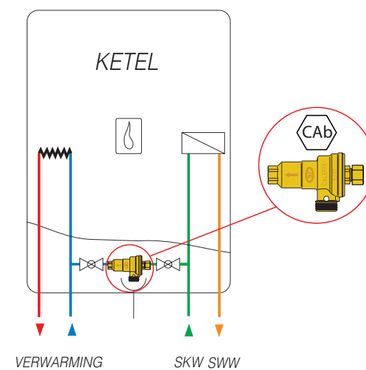
11. Vullen van wandketels voor alleen verwarming of verwarming en SWW zonder additieven (cat. 3)
