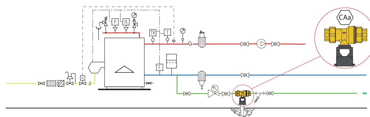
10. Vullen van verwarmingsinstallaties zonder additieven (cat. 3)
