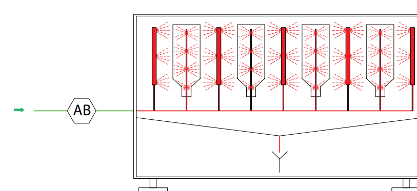
20. Wassen van melktanks (cat. 5)
