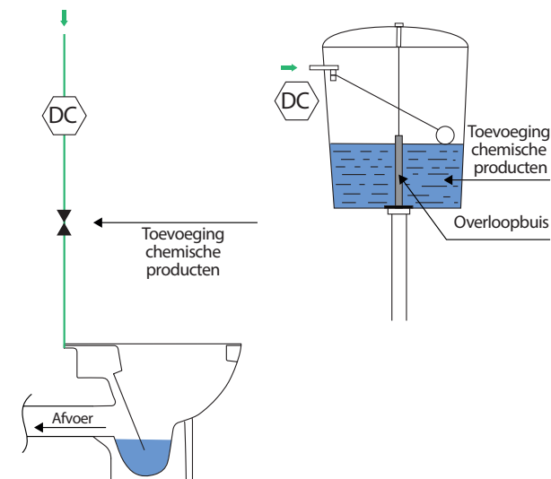
7. Spoelsysteem voor wc's en urinoirs met toevoeging van reinigingsmiddelen (cat. 5)
