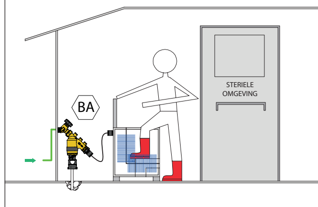
24. Laarzenwasinstallatie voor toegang tot beschermde gebieden (cat. 4)
