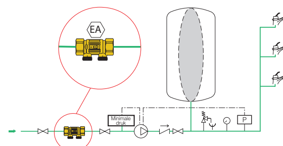
4. Hoge drukstations (cat. 2)
