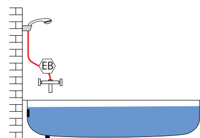
6. Handdouche die is aangesloten op de kranen voor badkuip, wastafel, met uitzondering van wc en bidet (cat. 5)
