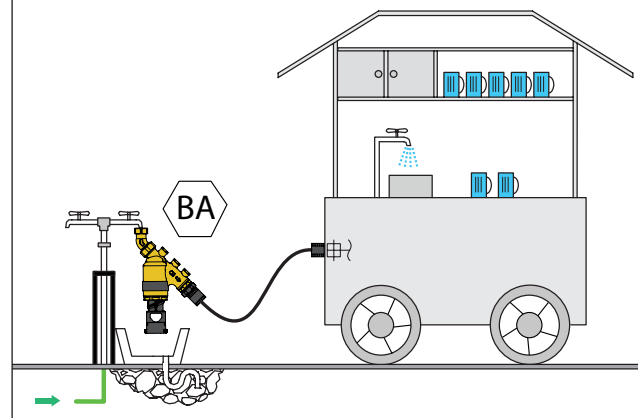
25. Aansluiting op mobiele stands en recreatiegebieden (cat. 4)
