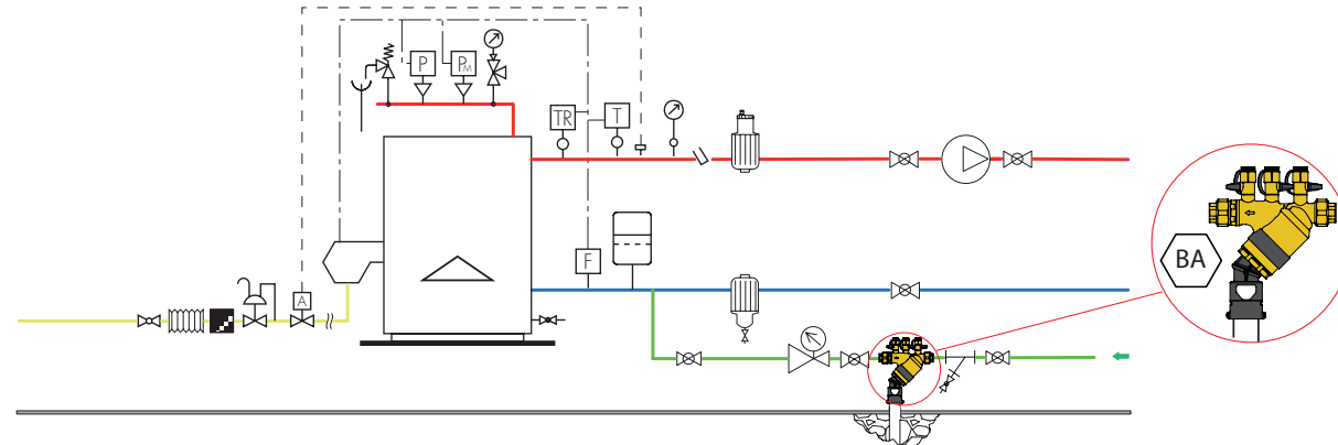
13. Vullen van verwarmingsinstallaties met additieven (cat. 4)
