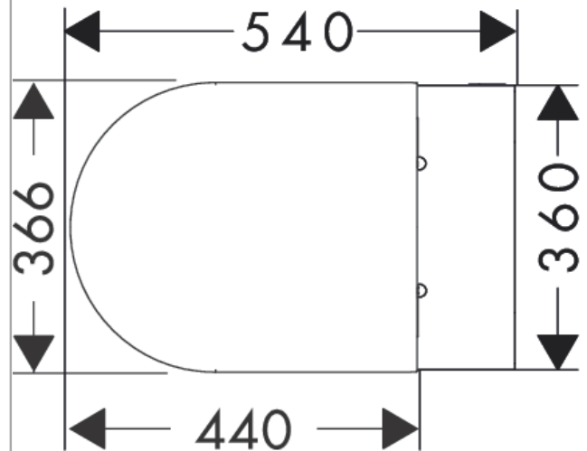
Maattekening
