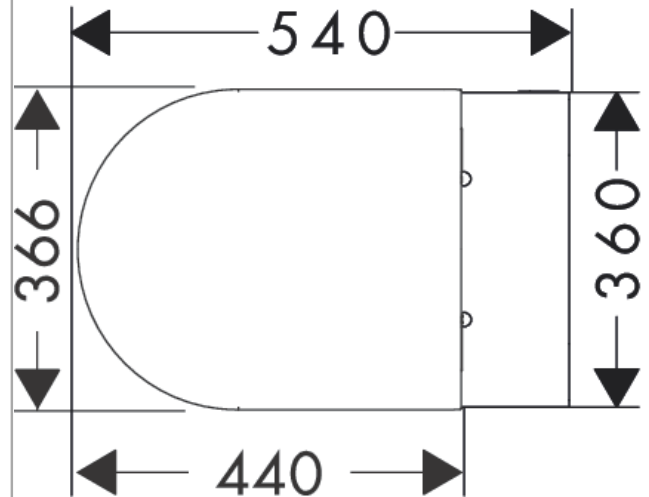
Maattekening
