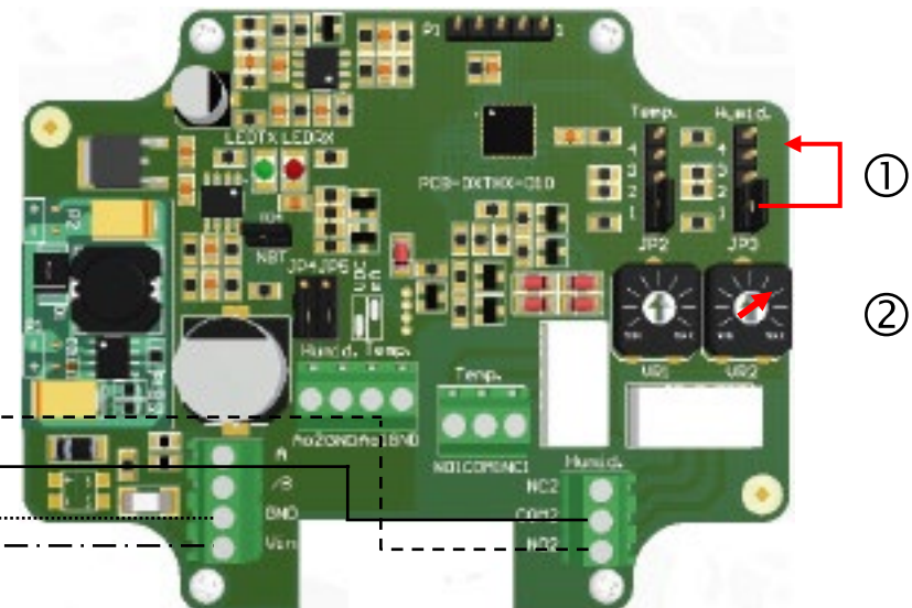
Printplaat Vocht kanaalopnemer
