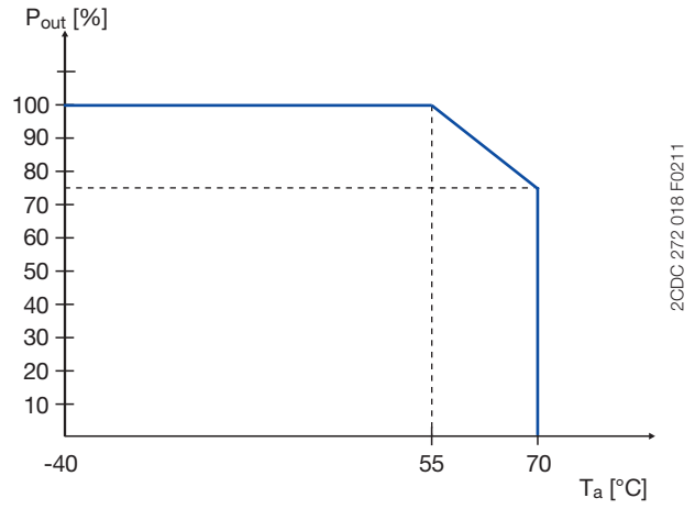
CP-E 24/20.0, CP-E 48/10.0
