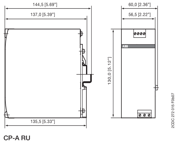
CP-A RU
