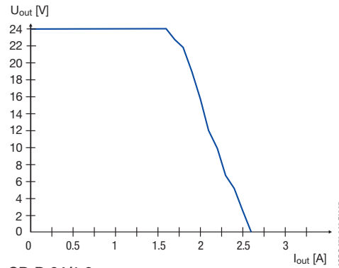
CP-D 24/1.3
