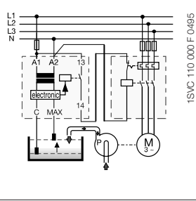
CM-ENE MAX
