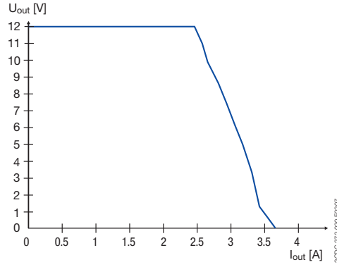
CP-D 12/2.1
