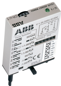
CR-U T
