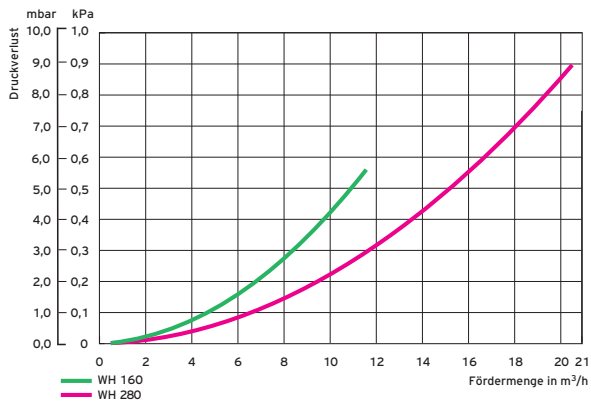
Hydraulische Weiche WH 160 und WH 280
