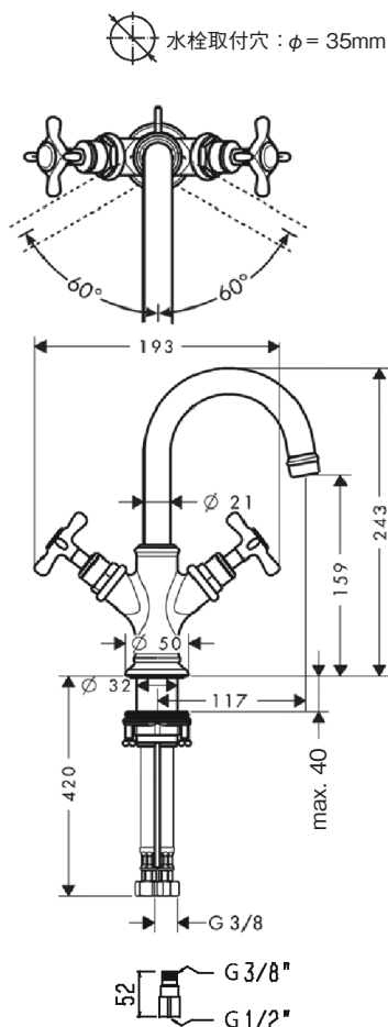
完成図
