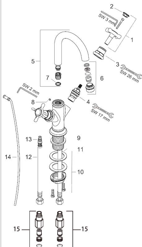
部品リスト
