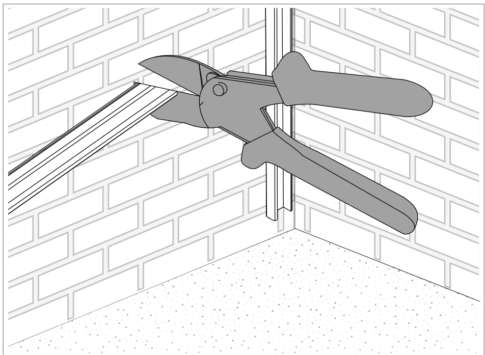
Fig. 4: Mitre cuts: Cutting the WDK mini trunking
