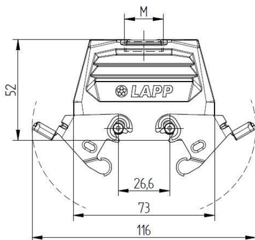
Kabeleingang gerade
