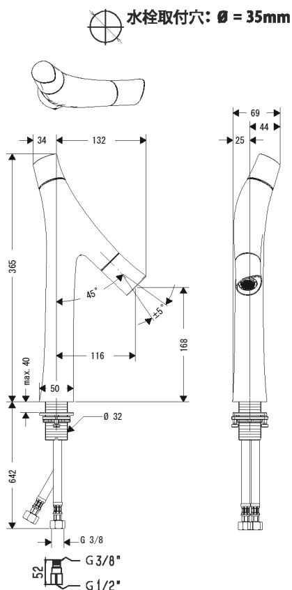
完成図
