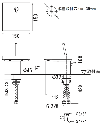
完成図
