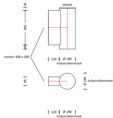
kanaal met roosterbox 400 x 100
