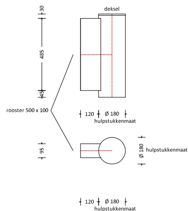
kanaal met roosterbox 500 x 100
