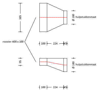
rechte roosterschoen 400 x 100
