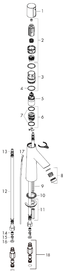
製品分解図
