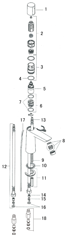
製品分解図
