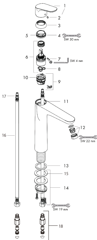
製品分解図
