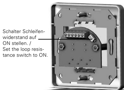
Ansicht RCM-A Modul nach dem Öffnen
