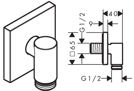
FixFit Fine E 28883XX0 / 28883XX7
