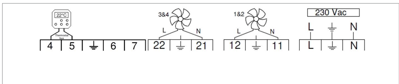
Figuur 23 - Hoofdaansluitingen voor de installatie
