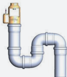
Afbeelding 1: KHS vrije uitloop met overloopbewaking en sifon
