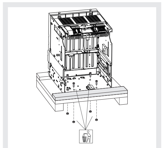
Figura 14 Parte fija UL
