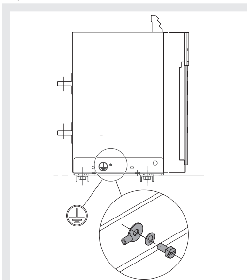
Figura 73 - Ejecución fija
