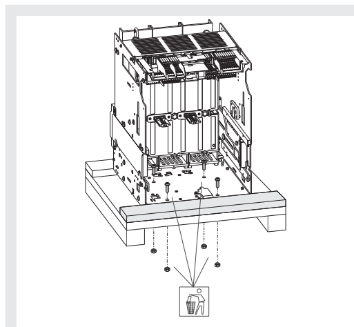
Figura 13 Parte fija IEC
