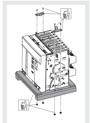
Figura 12 Parte móvil UL
