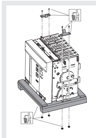
Figura 11 Parte móvil IEC
