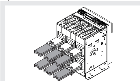
Figura 70 UL
