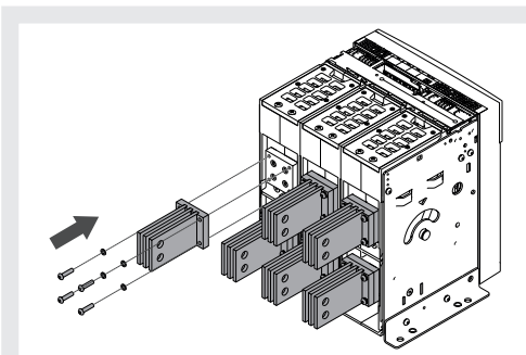
Figura 68 UL
