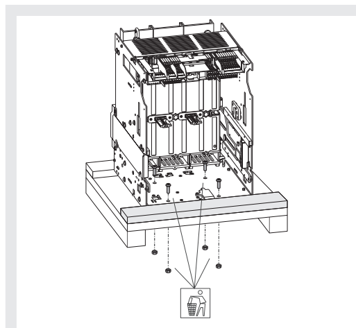
Figure 13 Partie fixe IEC
