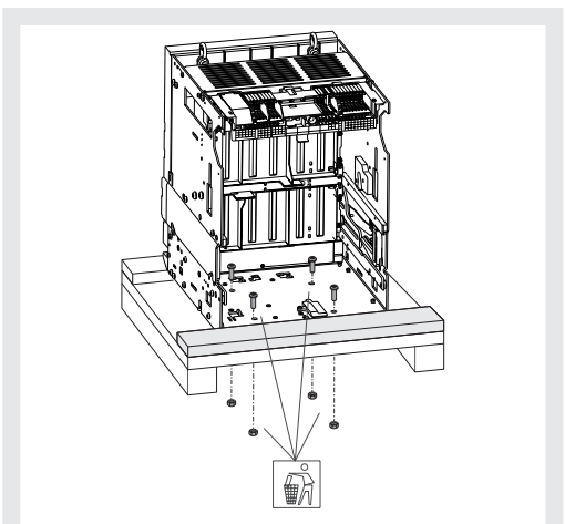
Figure 14 Partie fixe UL
