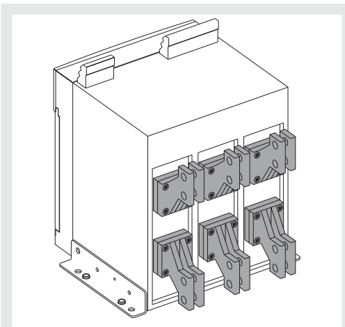
Figure 60 SVR - Arrière verticales épanouies IEC (E2.2)
