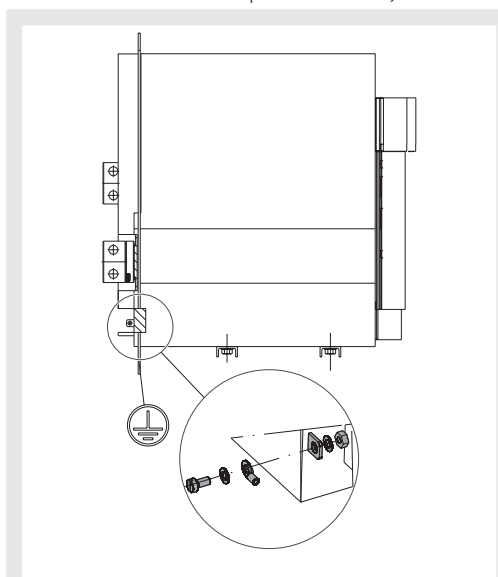
Figure 74 - Version débrochable
