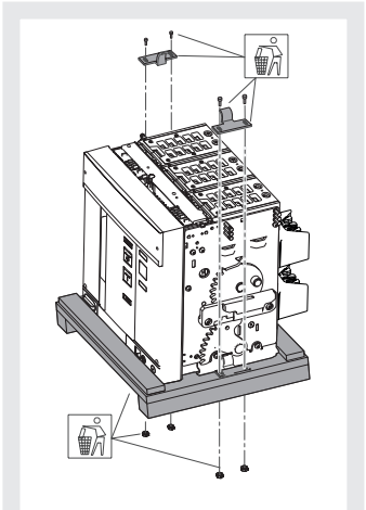
Figure 12 Partie mobile UL
