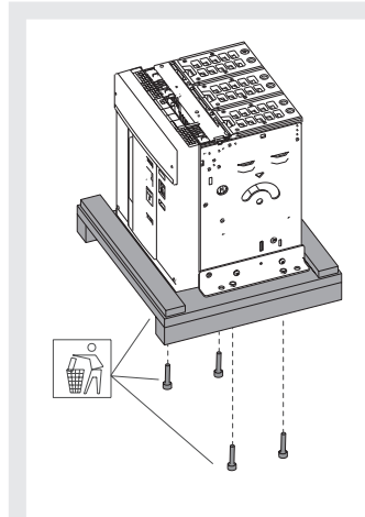
Figure 10 Disjoncteur fixe
