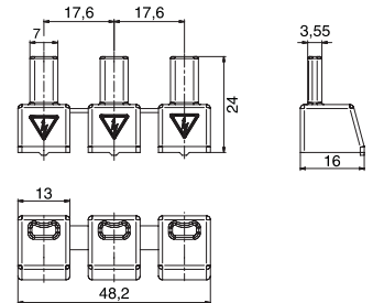
ZV-BS-UL
