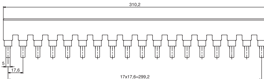
Z-SV/UL-16/TE/18
