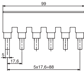
Z-SV/UL-16/TE/6
