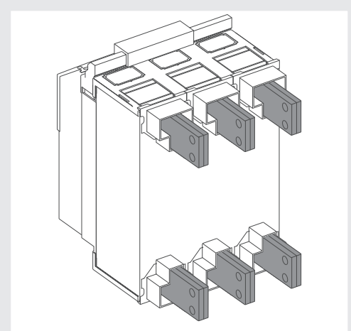
Abbildung 59 - F - VR - Rückseitig vertikal UL Listed
