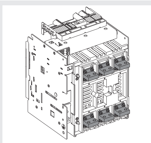
Abbildung 52 - W - HR - Rückseitig horizontal IEC
