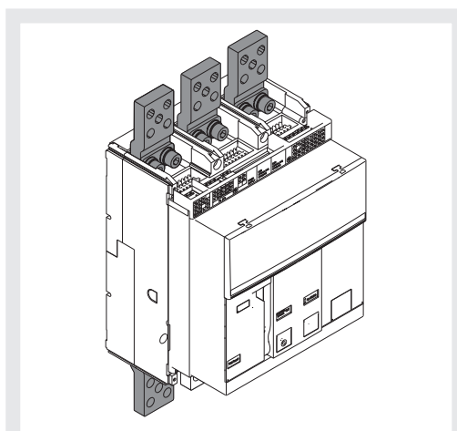
Abbildung 49 - F - EF - Vorderseitig verlängert IEC-UL
