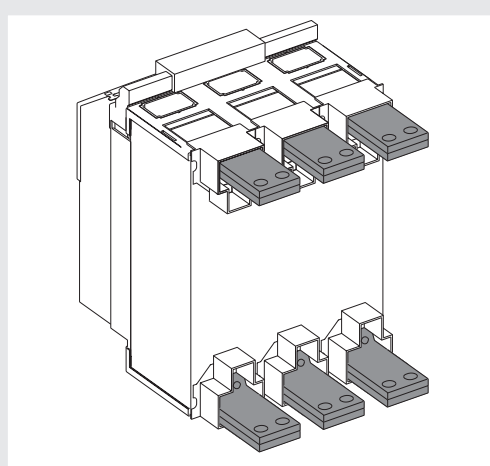
Abbildung 58 - F - HR - Rückseitig horizontal UL Listed
