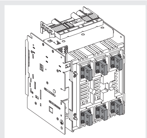
Abbildung 53 - W - VR - Rückseitig vertikal IEC
