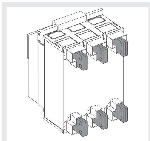
Abbildung 47 - F - VR - Rückseitig vertikal IEC
