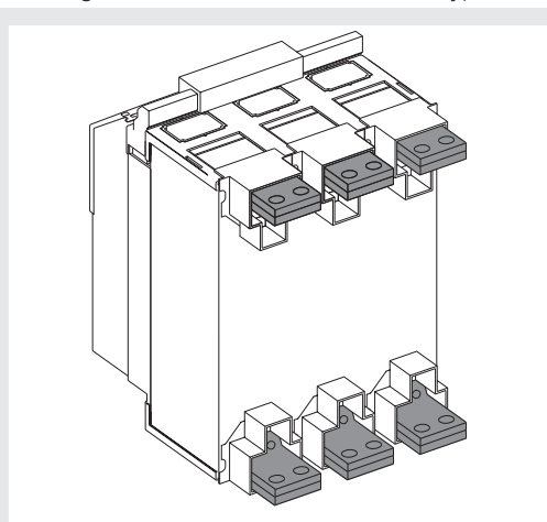
Abbildung 46 - F - HR - Rückseitig horizontal IEC
