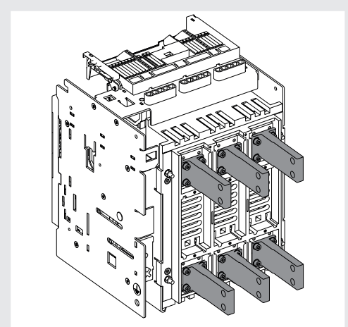
Abbildung 61 - W - VR - Rückseitig vertikal UL Listed
