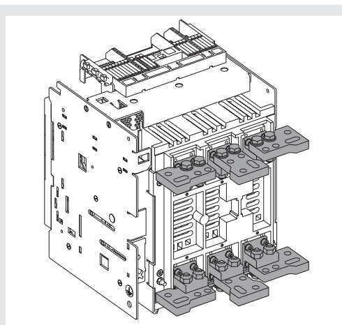
Abbildung 54 - W - SHR - Rückseitig V-förmig horizontal IEC
