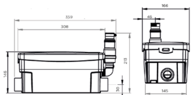
Afmetingen (mm)
