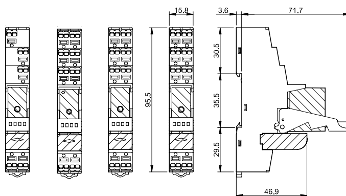
Type 48.P8 2 wisselcontacten 10 A 250 V AC1
