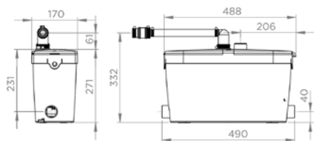
Afmetingen (mm)
