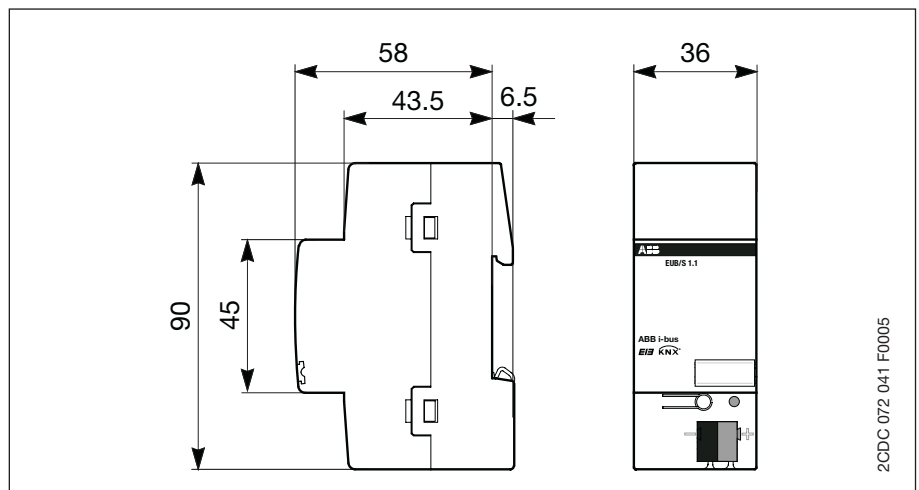
Abb. 3: Gerätemaße
