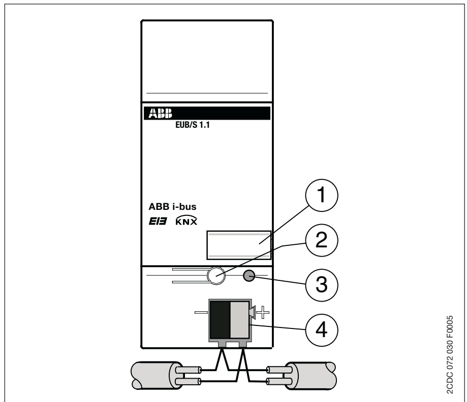
Abb. 2: Anschlussbild
