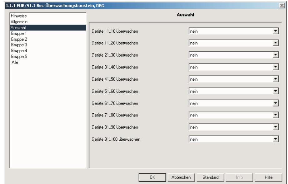
Abb. 5: Parameterfenster „Auswahl“
