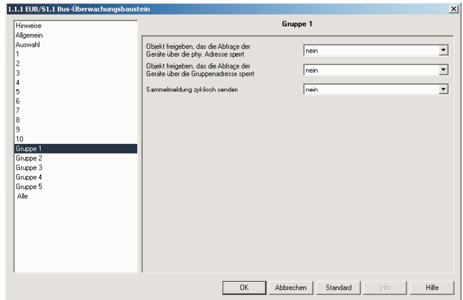
Abb. 11: Parameterfenster „Gruppe 1...5“
