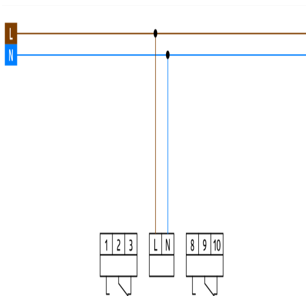
Schakelschema
