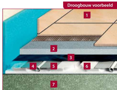
Opbouw voorbeeld (ex. vloerplaat en vloerafwerking)
