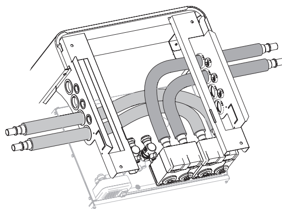
CONFIGURATIE 4 | Cv rechts + Bron links
