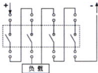
DC500V 4极串联
