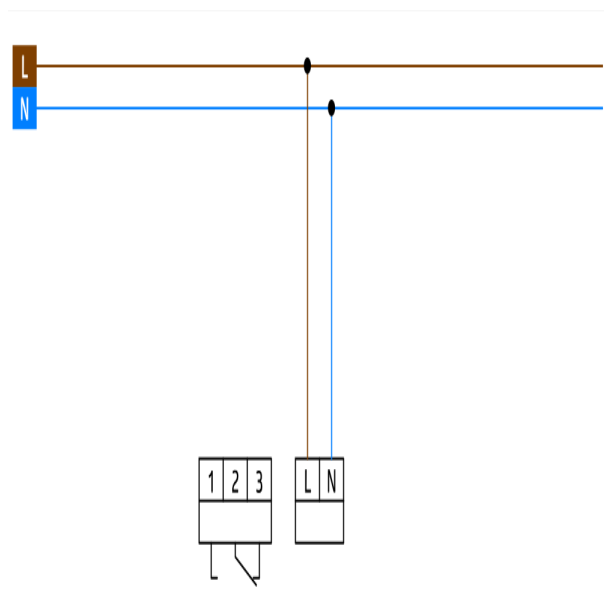
Schakelschema
