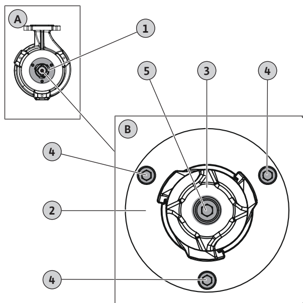
Fig. 9: Výměna mělnícího zařízení
