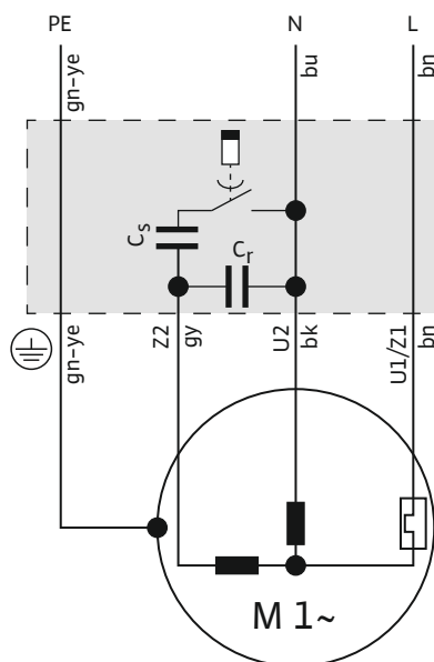
Fig. 6: Schéma zapojení 1~ motoru
