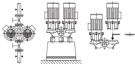
Fig. 2: Ansicht Atmos GIGA-D
