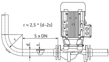
Fig. 9: 펌프 전단 및 후단의 안정화 구간
