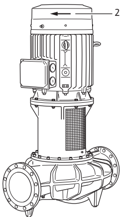
Fig. 12: 회전방향 점검
