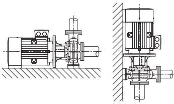
Fig. 3: Ansicht Atmos GIGA-B
