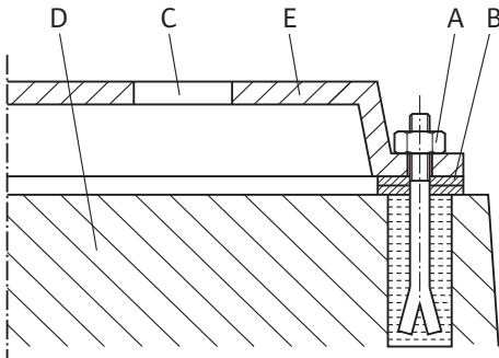
Fig. 8: 기초 나사 연결부 예시
