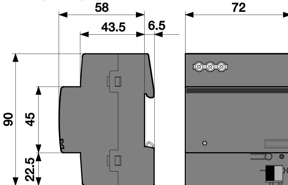
Abb. 2: Abmessungen 6201/640.1
