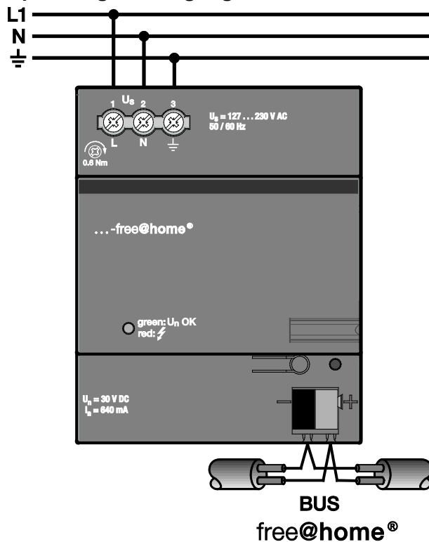
Abb. 3: Elektrischer Anschluss 6201/640.1
