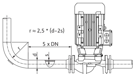
Fig. 9: Διαδρομή ηρεμίας πριν και μετά την αντλία
