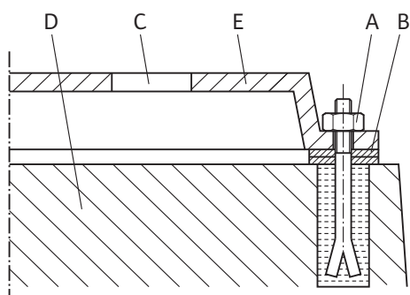
Fig. 8: Παράδειγμα για κοχλίωση θεμελίωσης
