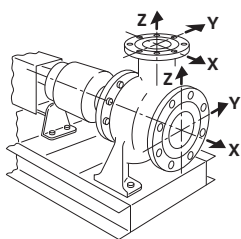
Fig. 6: Συνθήκες φορτίου 1A
